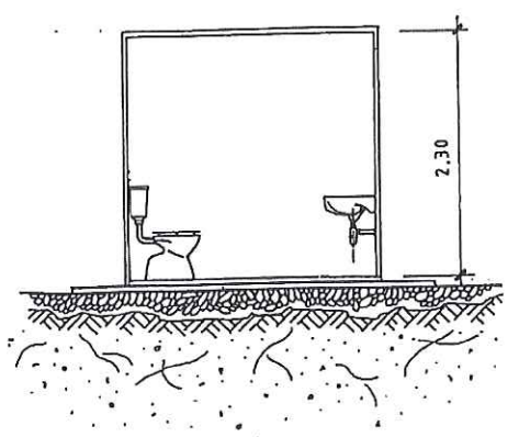
SEZIONE
